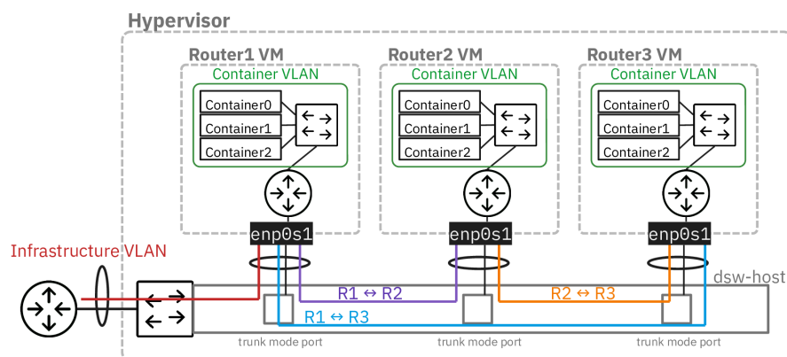
Topologie physique en étoile
