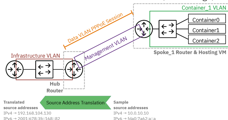
Traduction d'adresses sources pour les flux sortants du routeur Hub .
